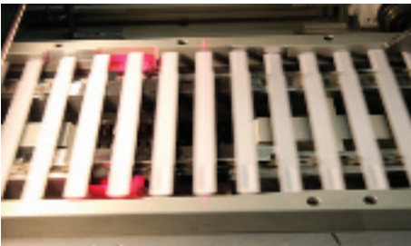
Med kameraoptik kollar man varenda sticka som rusar förbi. T ex längd och böjning.
